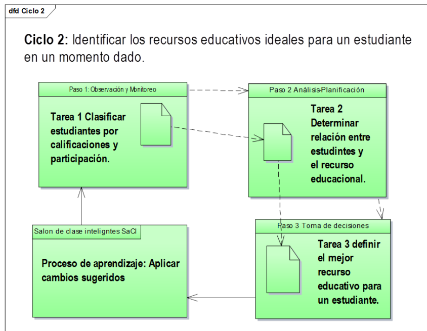
Figura 3.3: Esquema conceptual de Ciclo 2.
