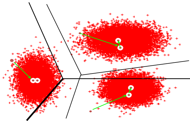
Clusterización Algoritmo K-Means
