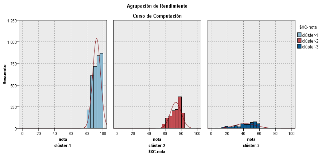
Figura 5.2: Agrupamiento K-Means del curso de computación.
