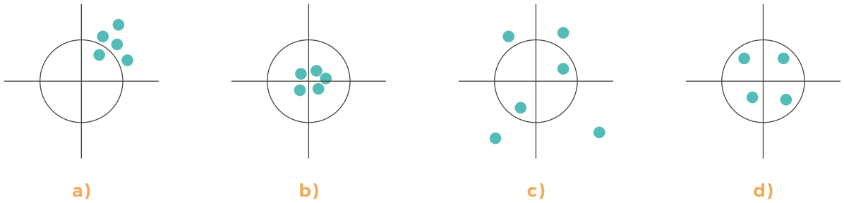
Figura 3 Diferencia entre precisión y exactitud. En a) y b) la precisión es elevada, mientras que en c) y d) es baja. Por su parte, en a) y c) la exactitud es baja, siendo alta en b) y d) . Fuente: Extraído de Olaya, 2012
