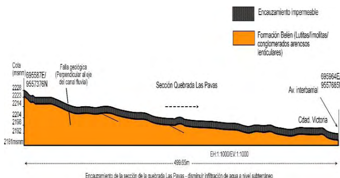
Fig. 16. Sección aproximada del encauzamiento de la quebrada Las Pavas.
