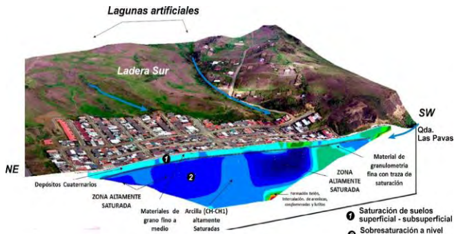
Fig. 10. Tomografía línea 2 transversal a la dirección del flujo superficial de "Ciudad Victoria".
