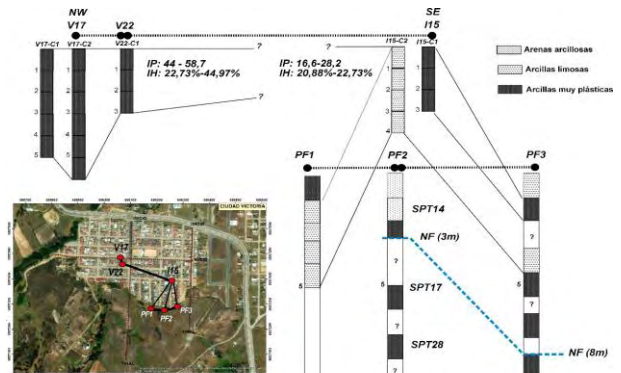
Fig. 9. Correlación de tipos geomecánicos de suelo de la zona urbana de Ciudad Victoria.
