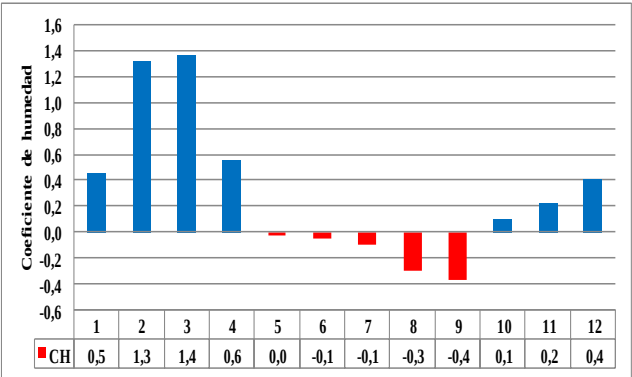
Fig. 4. Balance hídrico – coeficiente de humedad para el periodo 1960 – 2013.
