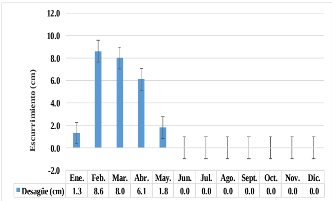
Fig. 5. Escorrentía pluvial o desagüe para ciudad Victoria y sus zonas aledañas. Estación la Argelia AP210. Periodo 1960 – 2013. (INAMHI, 2017)
