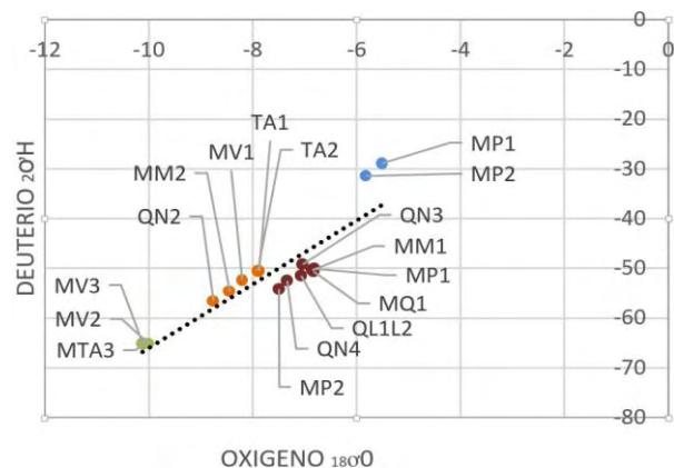
Fig. 12. Distribución del muestreo geoquímica de agua para análisis isotópico
