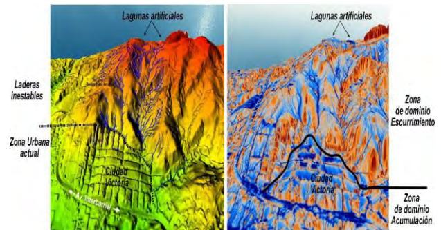
Fig. 2. Imágenes (DEM) del sector de Ciudad Victoria y su área de influencia, podemos reconocer las zonas de escurrimiento y acumulación dominantes de agua.
