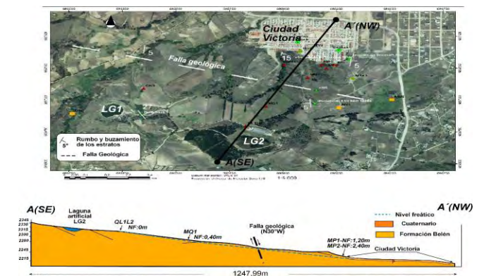
Fig. 8. Cortes geológicos (B-B'), donde se muestra la Formación Belén y la dirección de los estratos de rocas.
