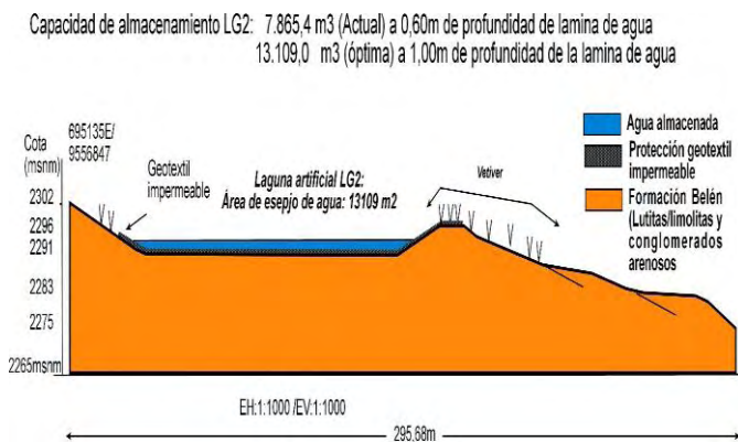
Fig. 15. Sección topográfica aproximada de Laguna LG2.
