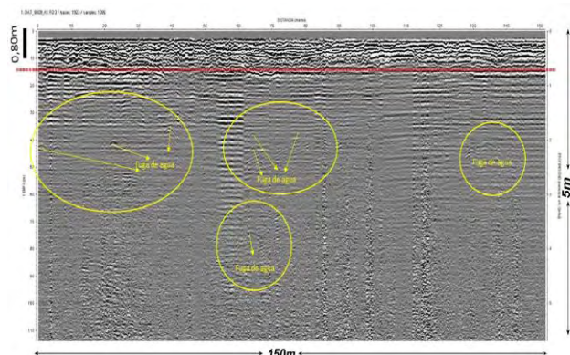
Fig. 11. Imagen de radargrama DAT_0409 levantado en la calle Clotario Maldonado de Ciudad Victoria
