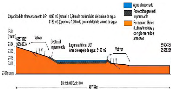
Fig. 14. Sección topográfica aproximada de Laguna LG1.
