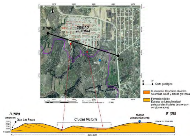
Fig. 7. Corte geológico (A-A') de la ladera sur de Ciudad Victoria.
