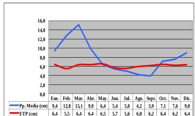
Fig. 3. Climograma de la estación La Argelia (AP210), comparación entre las variables precipitación media anual y evapotranspiración para el periodo 1960 – 2013.
