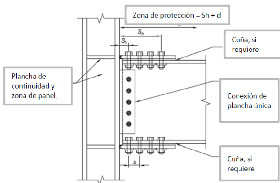
Figura 7. Esquema de conexión típica de tipo BFP adaptado de la normativa AISC/ANSI 358-16. Fuente: [5]
