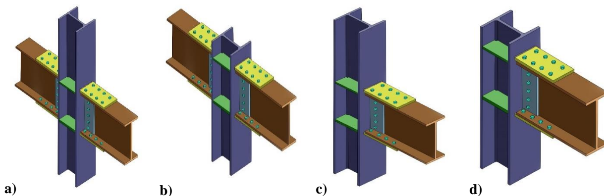
Figura 4. Diferentes tipos de nodos BFP: a) interno, b) interno último piso, c) de borde, d) de borde último piso
