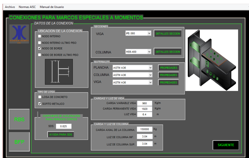
Figura 9. Interfaz gráfica para la recolección de datos, Ejemplo BFP
