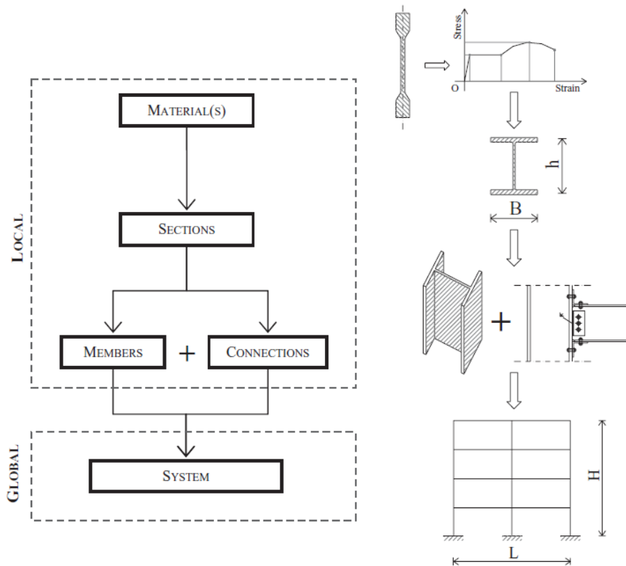
Figura 1. Relación jerárquica entre respuesta estructura local y global. Fuente: [2]
