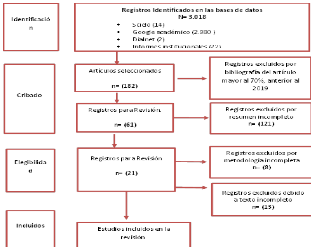
Figura 1. Flujograma Prisma
