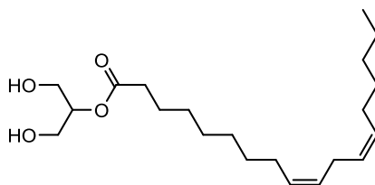
2-hidroxi-1-(hidroximetil)etil-9(Z),12(Z)-octadecadienoato (12)
