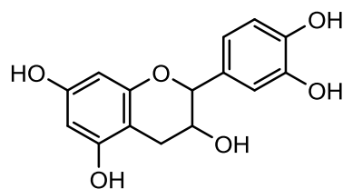
Catequina (23)
