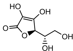
Ácido ascórbico (8)
