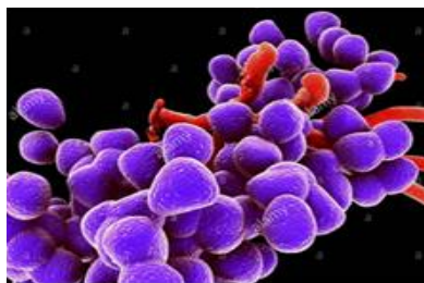
Figura 21. Enterococcus faecalis
