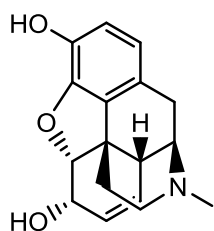
Morfina ( 18 )
