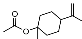
4-isopropenil-1-metilciclohexil acetato (16)
