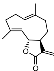
Germacranólidos ( 27 )
