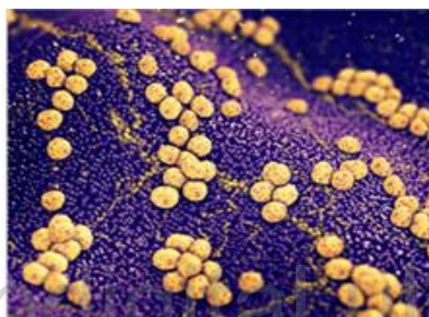
Figura 20. Staphylococcus aureus
