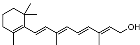
Vitamina A (7)
