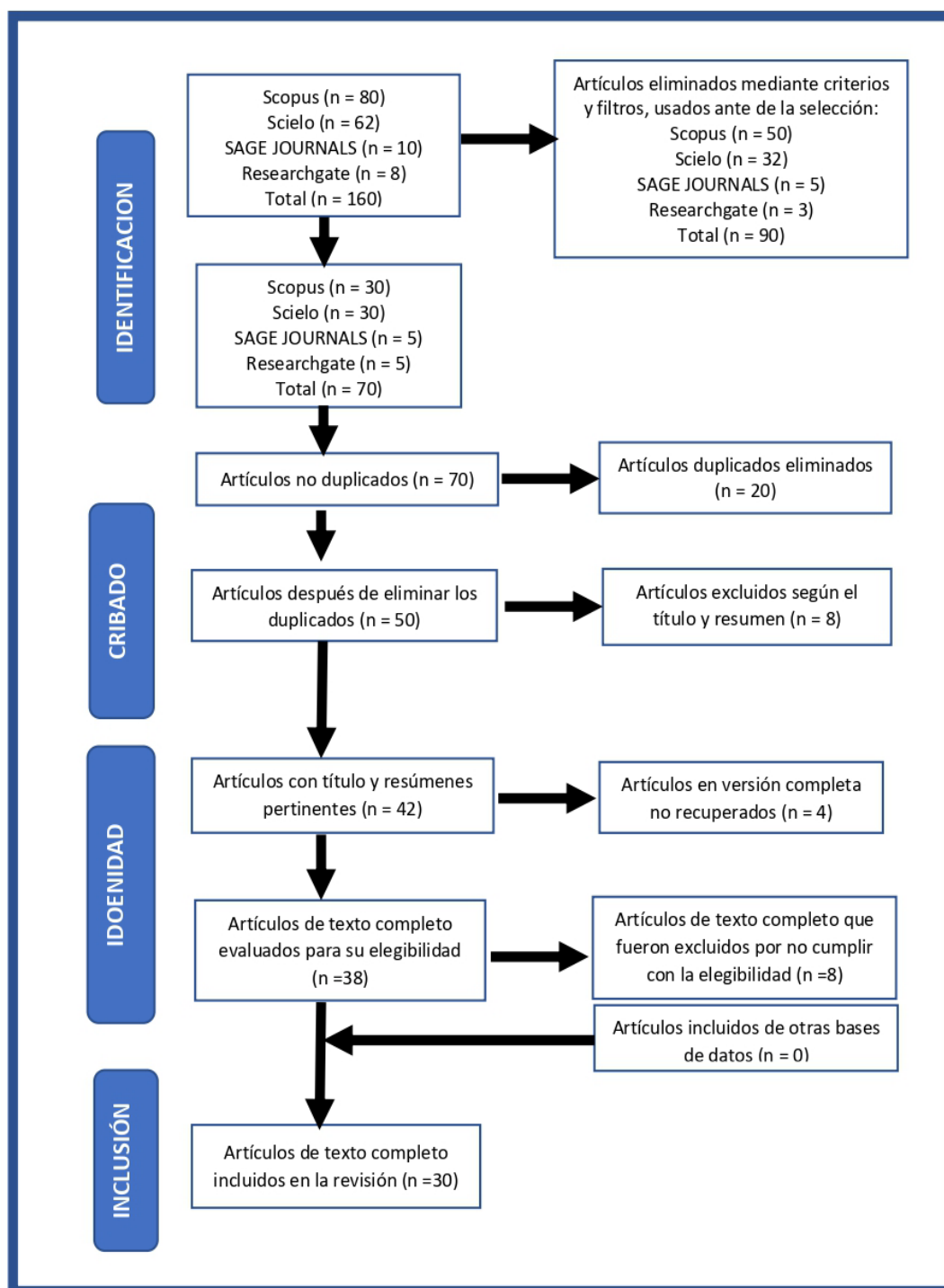
Figura 1: Flujograma PRISMA
