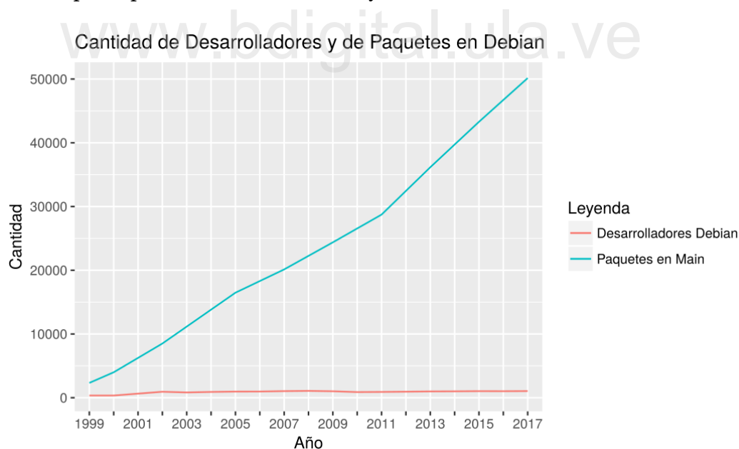
Figura 1.1: Crecimiento en el número de Desarrolladores Debian y paquetes del repositorio principal entre los años 1999 y 2017
