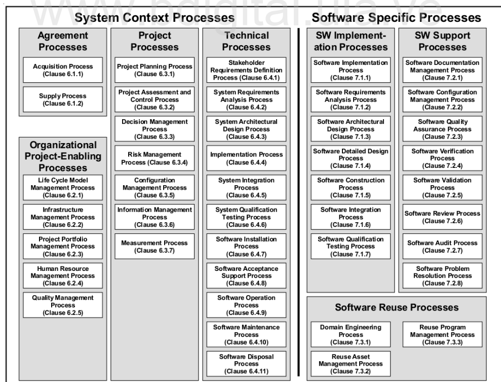
Figura 2.1: Grupos de los procesos del ciclo de vida
