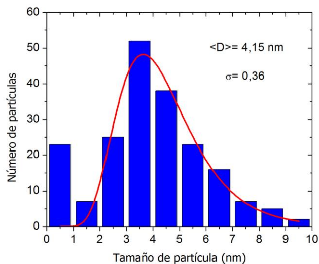
Fig. 5. Histograma de tamaños de partícula del nanocompuesto sintetizado.
