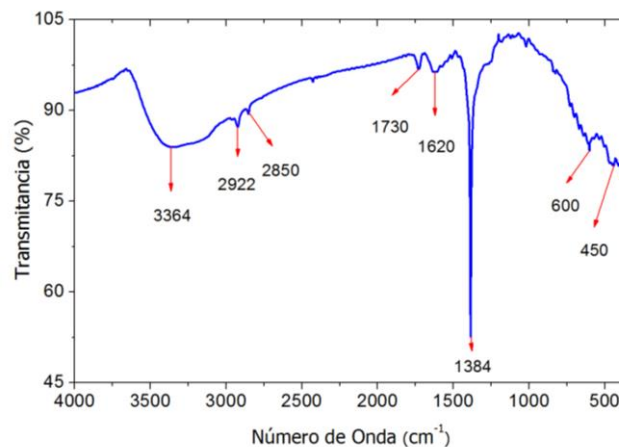
Fig. 3. Espectro FTIR del compuesto sintetizado.
