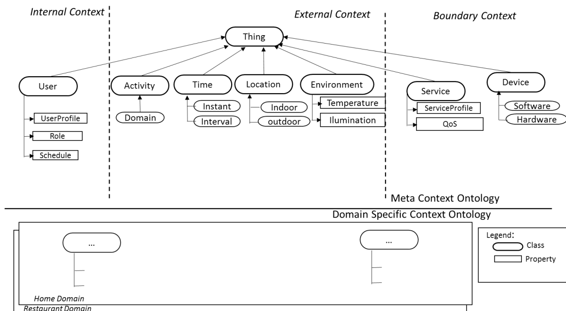
Figura 3.3: Modelo jerárquico de CAMEON (Fuente ?)
