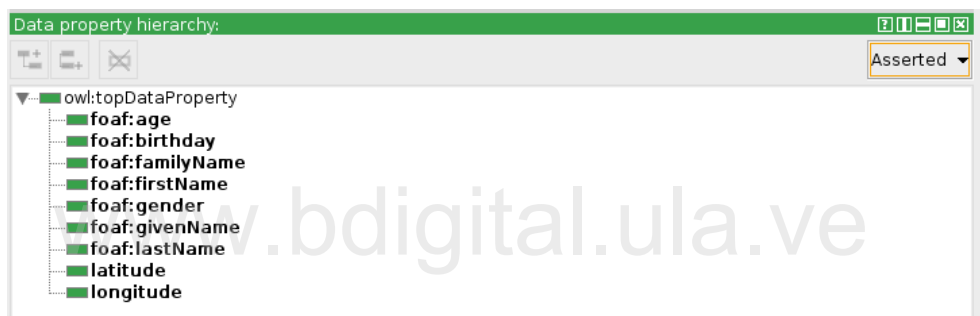
Figura 4.4: Propiedades de datos de CameOn en Protégé
