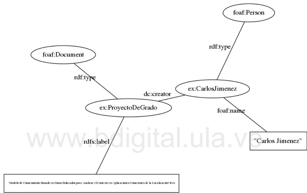
Figura 2.7: Grafo que representa las tripletas del ejemplo del la Figura ???
