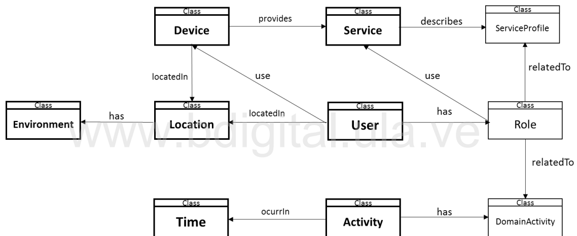
Figura 3.4: Relaciones entre las clases de CameOn (Fuente ?)
