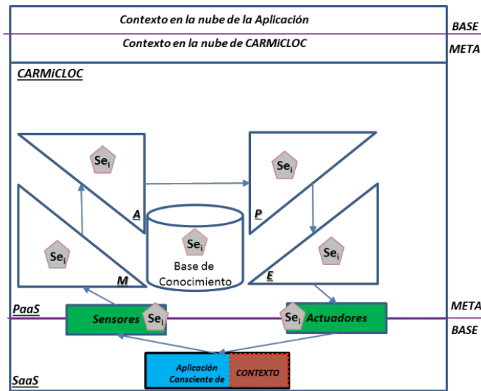
Figura 3.1: Arquitectura de CARMiCLOC (Fuente ?)
