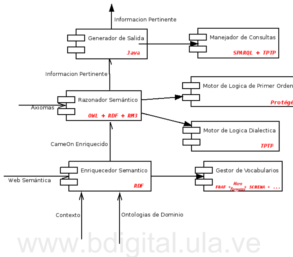
Figura 4.2: Arquitectura propuesta del Sistema con las tecnologías usadas
