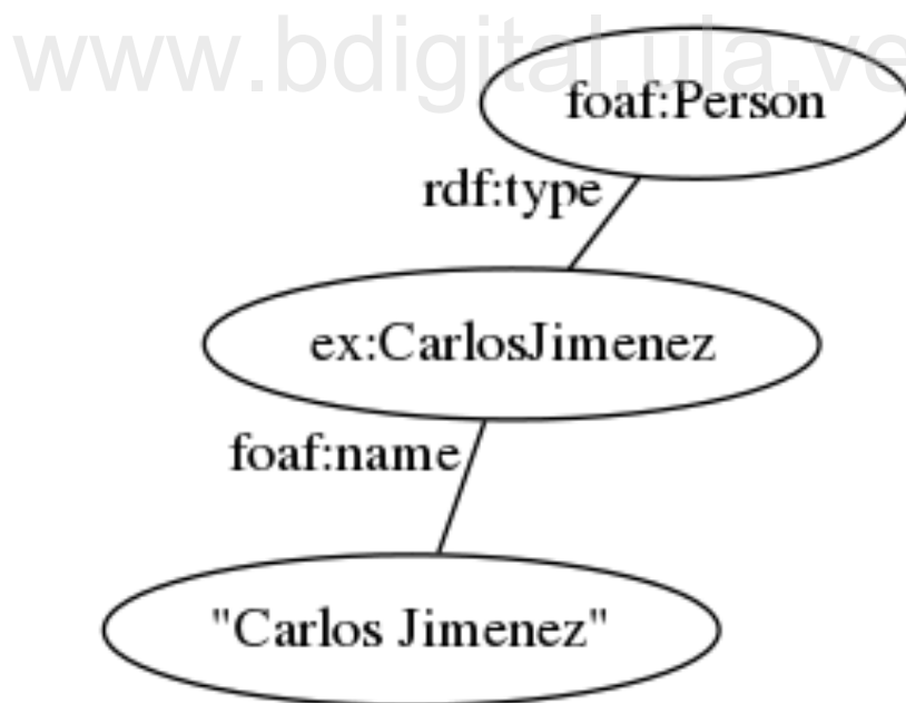
Figura 2.3: Grafo que representa las tripletas del ejemplo de la Figura ??
