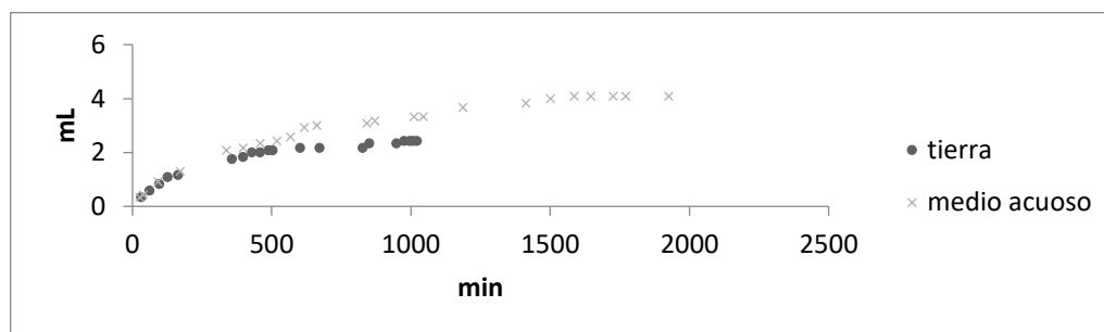
Figura 2. Tiempo de destilación de las raíces de vetiver en min vs. mL de AE obtenido
