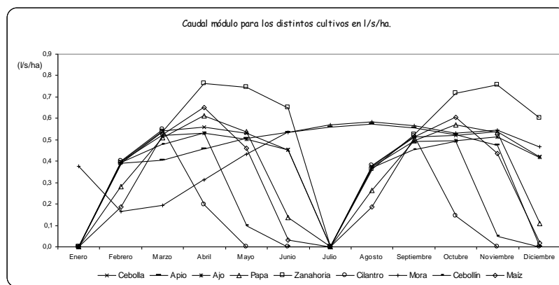
Figura 7. Curvas de caudal módulo para los diferentes cultivos en l/s/ha.
