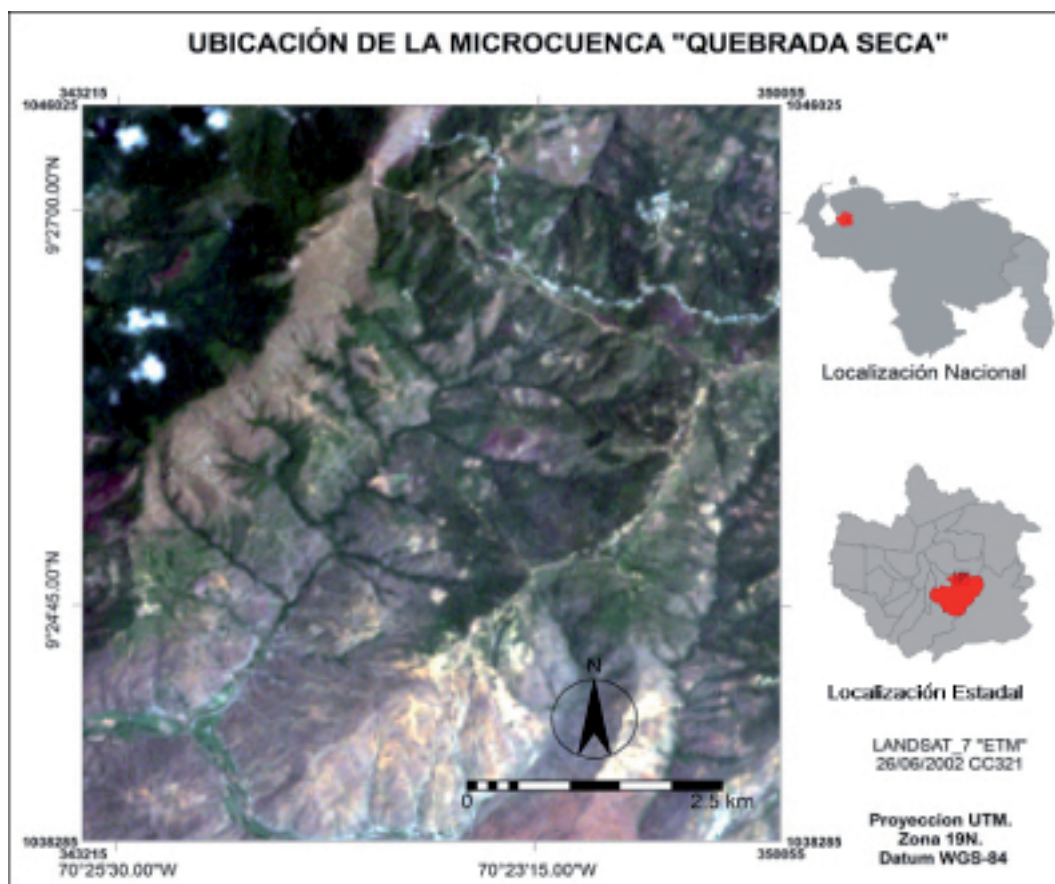
Figura 1.- Ubicación de la microcuenca quebrada Seca. Límite de la microcuenca superpuesto sobre una composición LANDSAT 7 ETM cc 321, del 26/06/2002, (landcover.org). Elaboración Propia.
