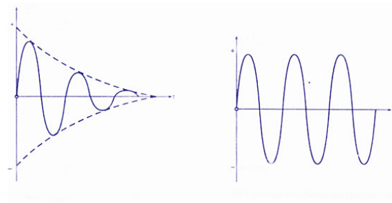
Figura 2.5: A la izquierda un ejemplo de oscilaciones en las cuales su fuente de energía interna expira y a la derecha con una fuente de energía interna infinita
