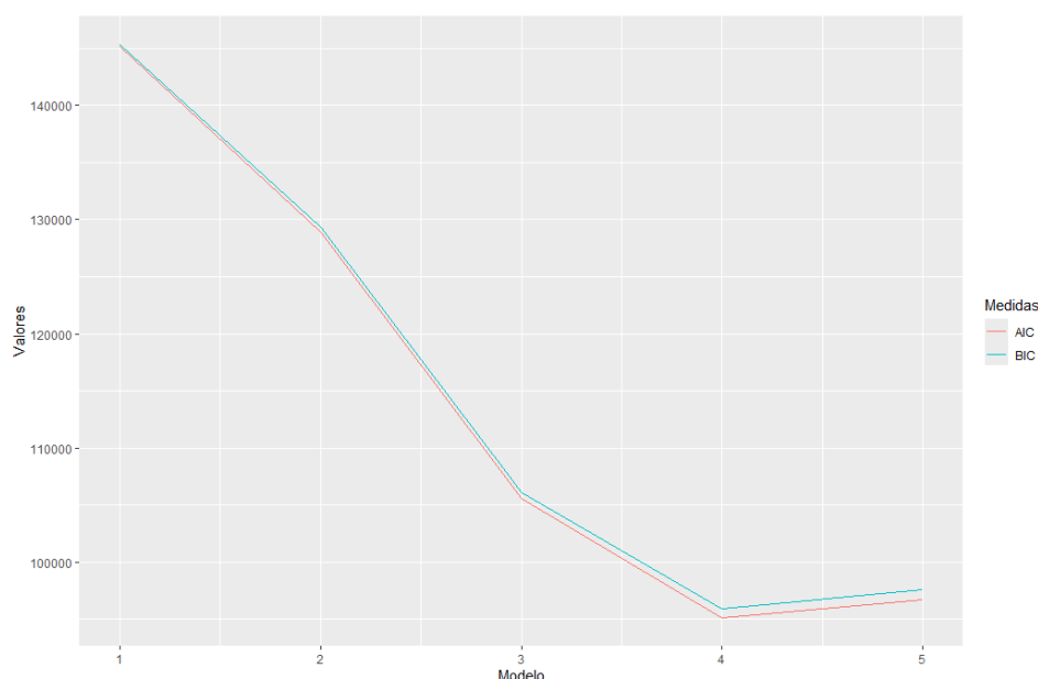
Figura 4. Valores de AIC y BIC para cada modelo de la dimensión situación migratoria
