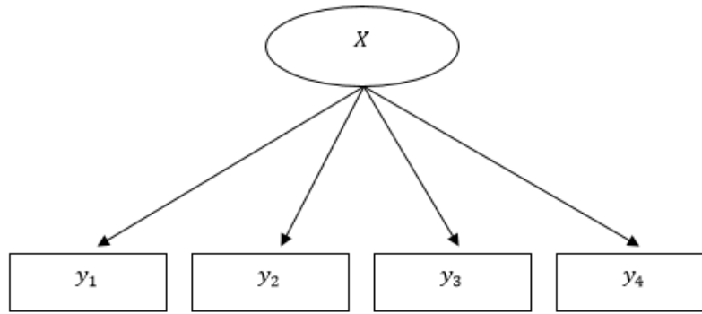
Figura 1. Representación gráfica de un modelo de clases latentes básico
