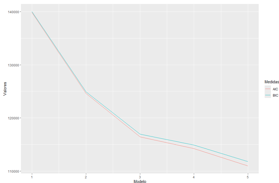
Figura 2. Valores de AIC y BIC para cada modelo de la dimensión sociodemográfica
