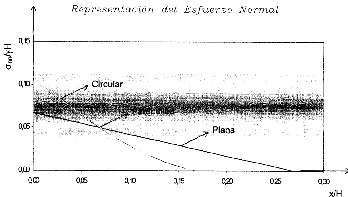
Fig. VI-9. Representación y comparación gráfica de \sigma_{nn}/\gamma H para las diferentes superficies de rotura (plana, parabólica y circular).
