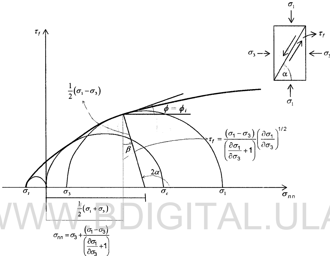
Fig. VI-2. Envolvente de rotura por cizallamiento en macizos rocosos. Tomado del manual de anclajes en Ingeniería Civil, Ucar (2004).
