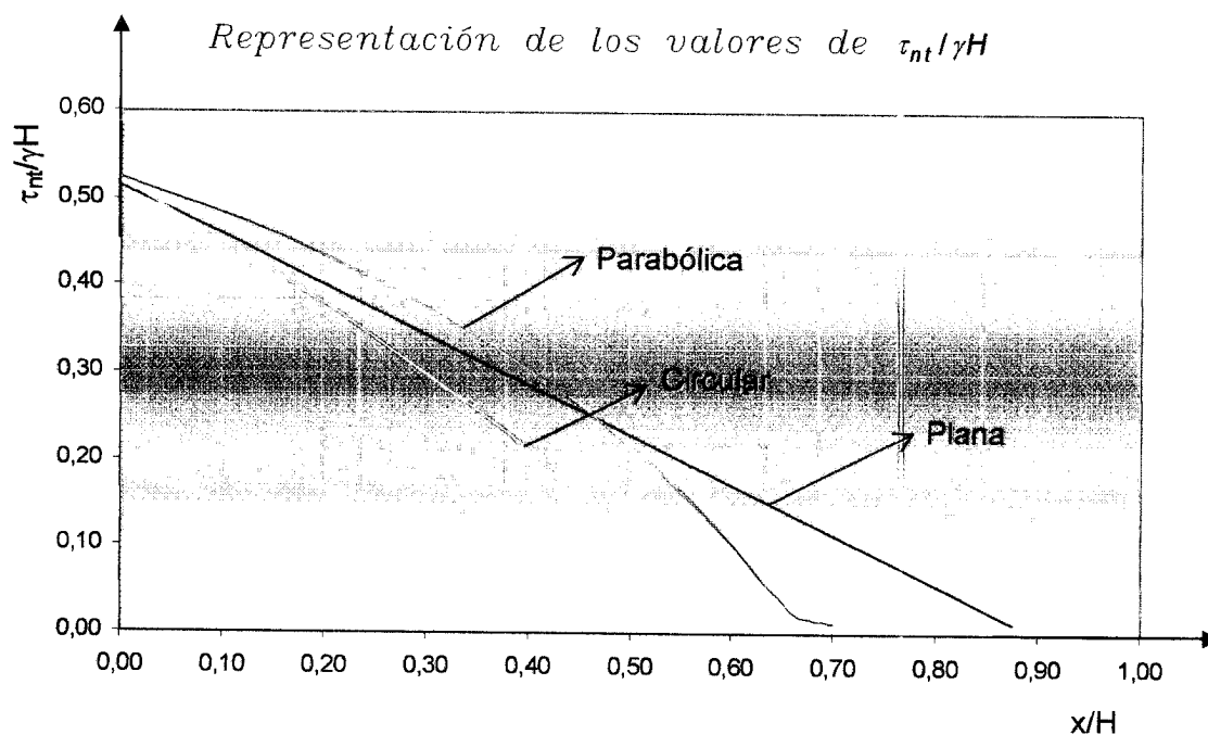
Fig. V-15 Representación y comparación gráfica de \tau_{nt}/\gamma H para las diferentes superficies de rotura (plana, parabólica y circular) para un talud inclinado.
