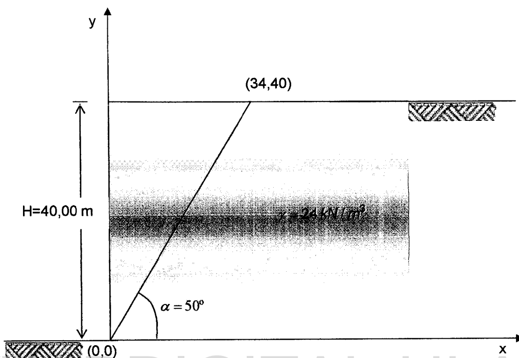
Fig. III-5 Representación gráfica de la superficie de rotura plana.
