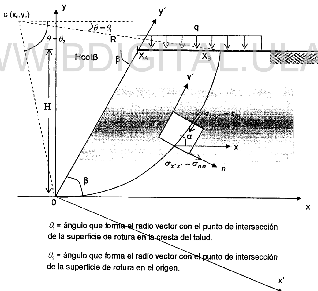
Fig. V-1 Representación de la superficie de rotura circular y sus relaciones geométricas.
