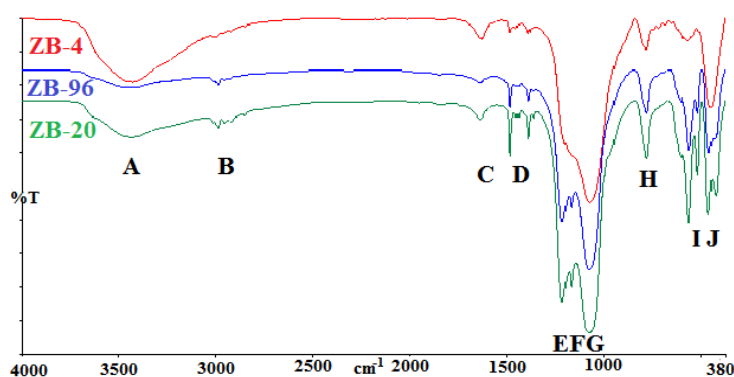
Figura 1. Espectro IR-TF de los materiales ZB-4, ZB-20 y ZB-96.
