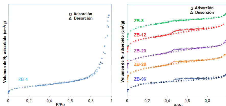
Figura 4. Isotermas de adsorción-desorción de N 2 obtenidas para los materiales en forma ácida.
