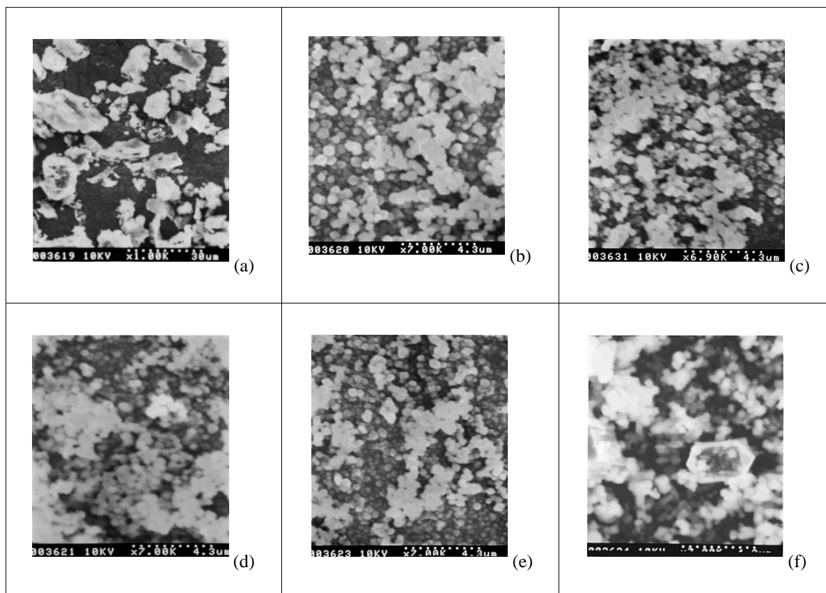
Figura 3. Micrografías de los materiales sintetizados por variación del tiempo de cristalización. (a) ZB-4, (b) ZB-8, (c) ZB-12, (d) ZB-20, (e) ZB-28 y (f) ZB-96.
