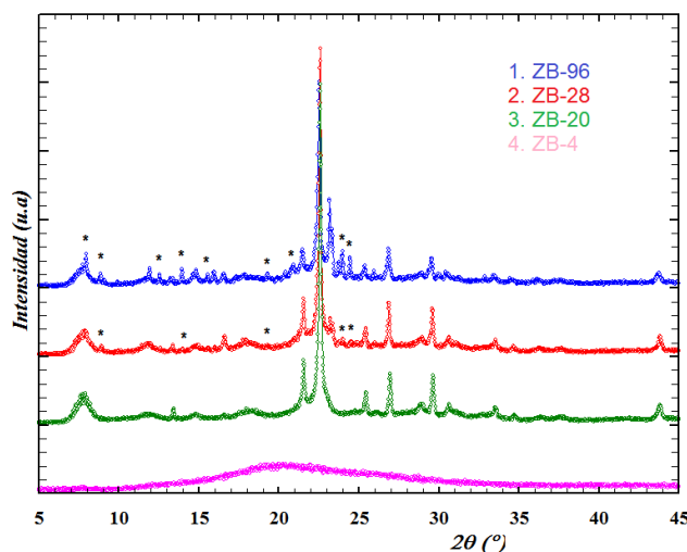
Figura 2. Patrón de difracción de los materiales sintetizados con tiempos de cristalización de 4, 20, 28 y 96 horas. (*) Rótulos de picos de difracción asociados con la fase de la zeolita MFI.
