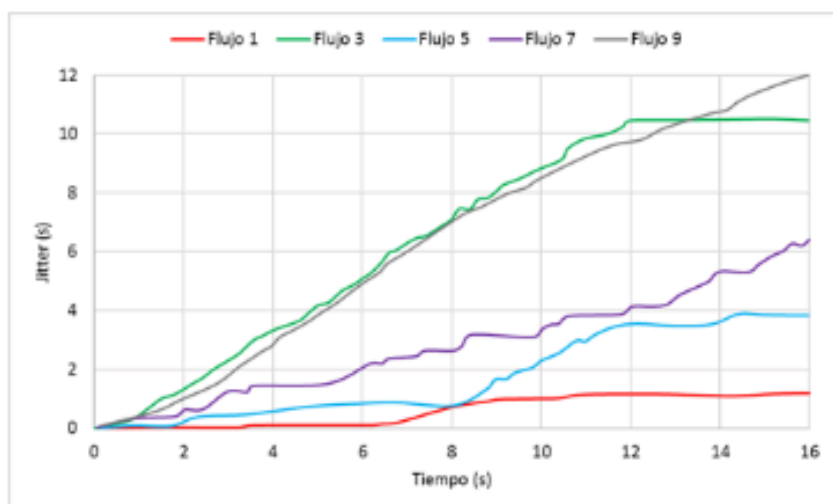
Figura 5 Suma del Jitter de los flujos, para cada uno de los escenarios
